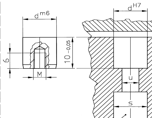
Senkung DIN 912
